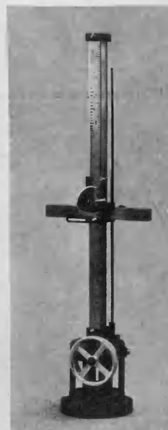
3. Дефлекторъ, приборъ для измѣренія магнитныхъ силъ, отклоняющихъ стрѣлку компаса. (См. Девиція.)
